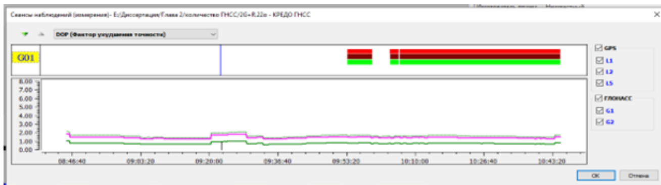
Рисунок 2.10 — Изменение p-dop фактора. ГНСС: ГЛОНАСС + GPS. T_{\text{изм.}} = 2 ч.
